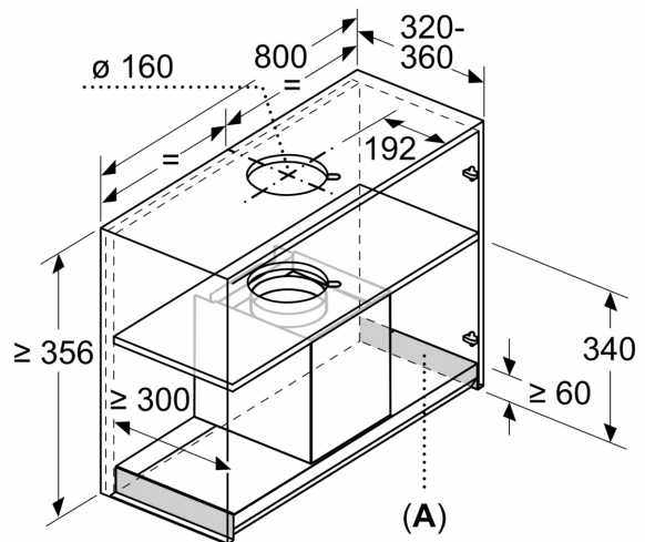
Dimensiuni în mm Model de montaj
