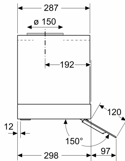
Dimensiuni în mm Vedere din lateral
