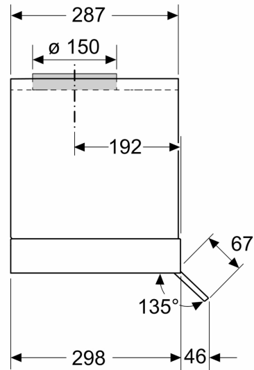
Dimensiuni în mm Vedere din lateral
