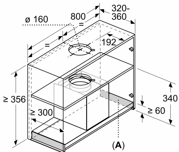
Dimensiuni în mm Model de montaj
