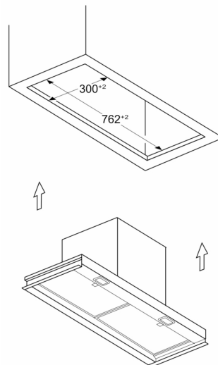
Dimensiuni în mm Exemplu de instalare în decupajul din mobilier
