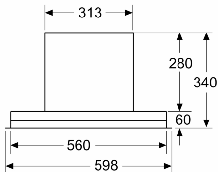
Dimensiuni în mm Vedere din față
