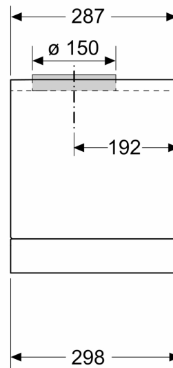
Dimensiuni în mm Vedere din lateral
