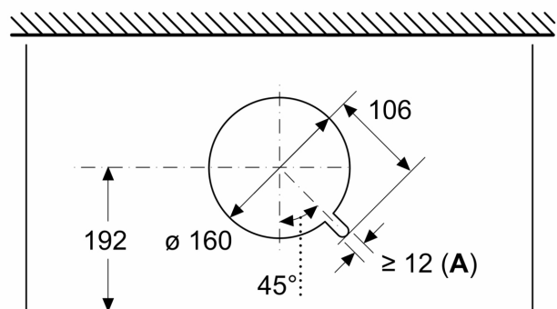
Dimensiuni în mm Vedere de deasupra
